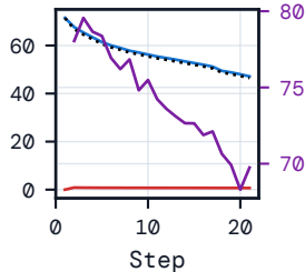
mRMR FCD
