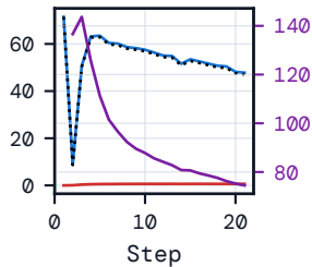
mRMR FCD
